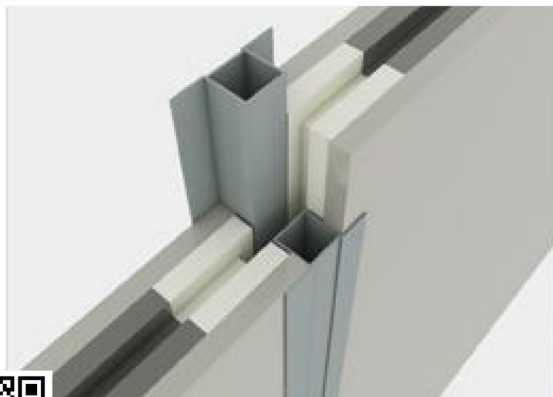
对夹式可拆隔墙搭接
