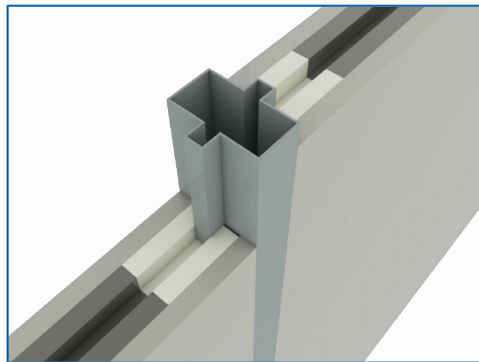
宽缝隔墙搭接
