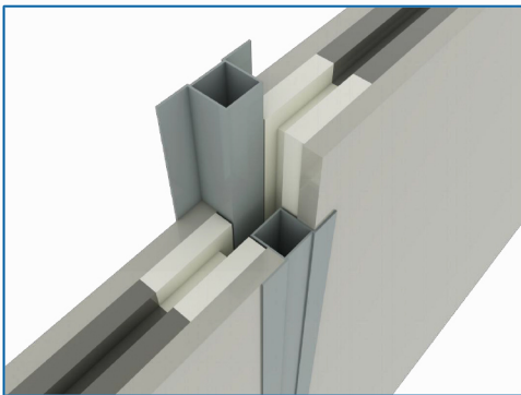
对夹式可拆隔墙搭接
