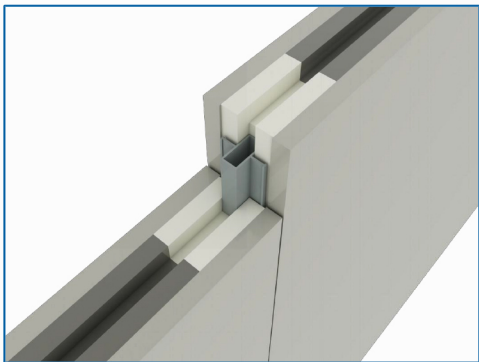
中置铝隔墙搭接
