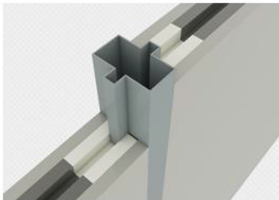
宽缝隔墙搭接
